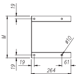
Corte K-K (Fixação do ventilador)
