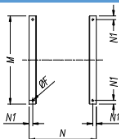
Corte K-K (Fixação do ventilador)
