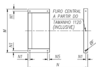
Corte K-K (Fixação do ventilador)
