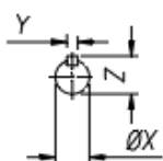
Ponta de eixo
