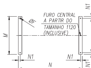
Corte K-K (Fixação do ventilador)
