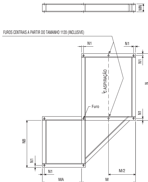
BASE ÚNICA POSIÇÃO "Y" PARA VENTILADORES COM POSIÇÕES A/0°, A/45°, A/90°, H/135°, H/180° e H/225°
