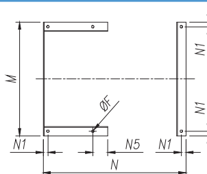
Corte K-K (Fixação do ventilador)
