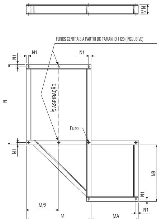
BASE ÚNICA POSIÇÃO "X" PARA VENTILADORES COM POSIÇÕES H/0°, H/45°, H/90°, A/135°, A/180° e A/225°
