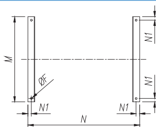
Corte K-K (Fixação do ventilador)
