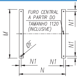
Corte K-K (Fixação do ventilador)
